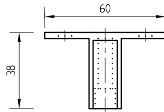
WKV 1 BAĞLAMA PAPUCU
