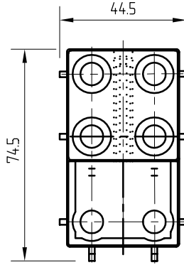
WKV 80 BAĞLAMA TAKOZU
