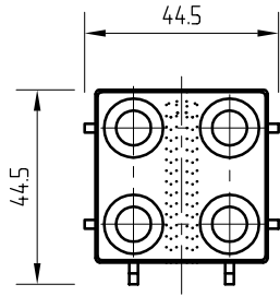
WKV 50 BAĞLAMA TAKOZU
