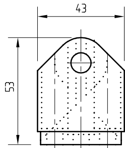
WKS 1 MAFSAL BAĞLANTISI
