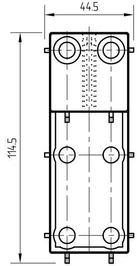
WKV 120 BAĞLAMA TAKOZU
