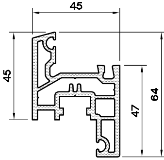
KANAT-45 PROFİLİ 1145.245
