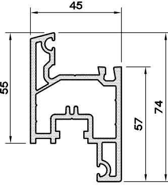
KANAT-55 PROFİLİ 1145.255
