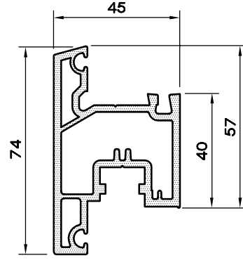
DİŞA AÇILAN KANAT-74 PROFİLİ 1145.274
