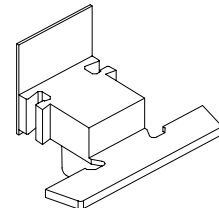
ORTAKAYIT UÇ KAPAMA PARÇ. E345.211
