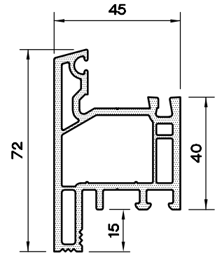
BİNİLİ KASA-72 PROFİLİ 1145.172
