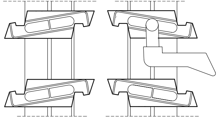
(SOL) (SAĞ) KEPENK MEKANİZMALI LAMEL ÇİTASI (H.- TK.) M331.376 - M331.380
