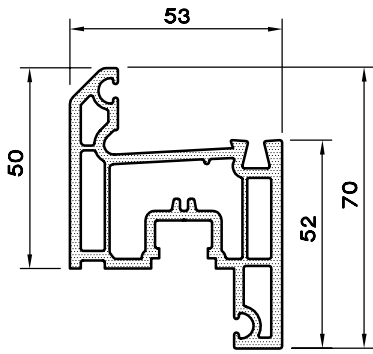
KANAT-50/3 PROFİLİ 1153.250
