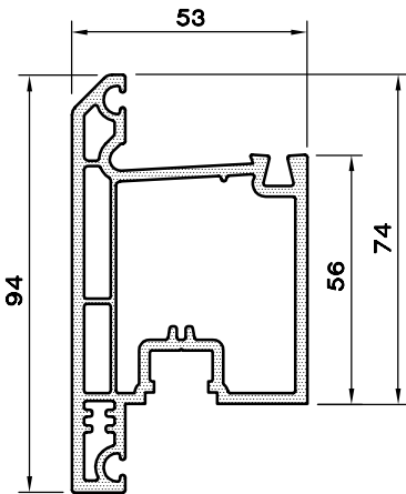
DIŞA AÇILAN KANAT-94/2 PROFİLİ 1153.494
