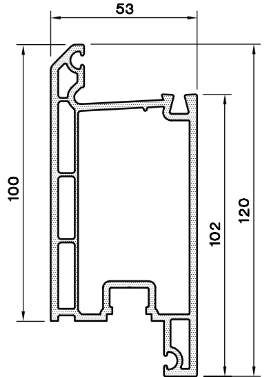
KAPI-100 PROFİLİ 1153.510
