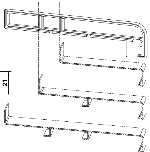
AL. DENİZLİK UÇ KAPAMA ( TAKIM ) E399.327
