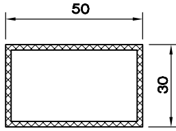
AL. KUTU PR. ( 30 X 50 ) 6199.135
