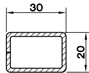
ORTAKAYIT -70/3 DESTEK SAÇI (30 X 20 X 2.0) 5160.332
