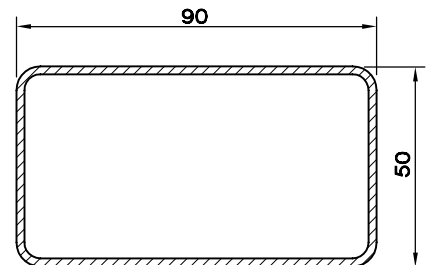
KUTU PR. (50 X 90 X 2.0) 5399.232
