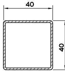
KUTU PR. (40 X 40 X 1.5) 5399.411
