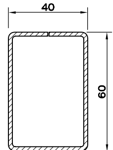
KUTU PR. (40 X 60 X 2.0) 5160.512
