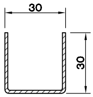
KASA -67 DESTEK SAÇI (1.5) 5160.111
