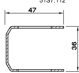
D.A. KANAT-96 DELİKLİ DES. SAÇI (1.5) 5260.421
