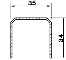
DAMLALIKLI KANAT -62 DESTEK SAÇI (1.5) 5160.241
