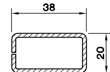
KUTU PR. (20 X 38 X 2.0) 5399.212
