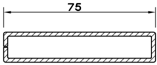
KUTU PR. (75 X 15 X 2.0) 5399.112
