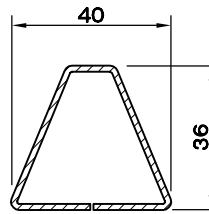
135° KÖŞE DÖNÜŞ DESTEK SAÇI (1.5) 5399.421
