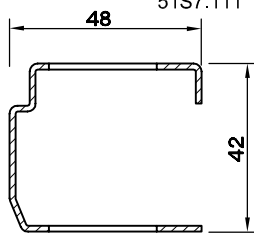
KANAT-76 DELİKLİ DES. SAÇI (1.5) 5260.411
