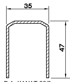
D.A. KANAT-96/3 DESTEK SAÇI (2.0) 5160.422
