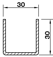
KASA -67 DESTEK SAÇI (2.0) 5160.112
