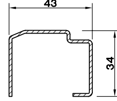
KANAT -62/2 DESTEK SAÇI (1.5) 5160.221
