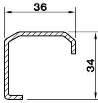
KANAT -62/3 DESTEK SAÇI (2.0) 5160.212
