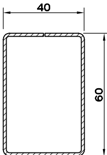
KUTU PR. (40 X 60 X 1.5) 5160.511
