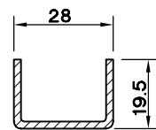
U PROFİLİ (2.0) 5199.111
