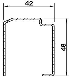
KANAT -76 DESTEK SAÇI (1.5) 5160.411
