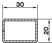
ORTAKAYIT -70/3 DESTEK SAÇI (30 X 20 X 1.5) 5160.331
