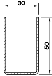
KASA -87 DESTEK SAÇI (1.5) 5160.121
