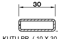
KUTU PR. (10 X 30 X 1.5) 5160.321
