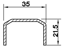
KANAT -50/3 DESTEK SAÇI (2.0) 5160.411
