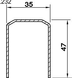
D.A. KANAT-96/3 DESTEK SAÇI (1.5) 5160.421
