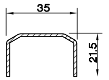
KANAT -50/3 DESTEK SAÇI (1.5) 5160.251
