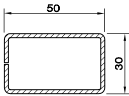
KUTU PR. (50 X 30 X 2.0) 5399.222
