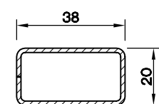
KUTU PR. (20 X 38 X 1.5) 5399.211
