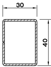
KUTU PR. (30 X 40 X 1.5) 5399.311
