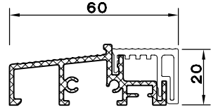
AL. EŞİK PR. 6399.103
