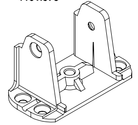
ORTAKAYIT-78/4 BAĞLAMA PARÇASI E161.136
