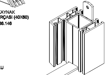
EŞİKSİZ KAPI LAMASI H399.211
