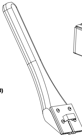
KAPI KAYNAK DESTEK PARÇASI SIKIŞTIRMA KOLU M669.111
