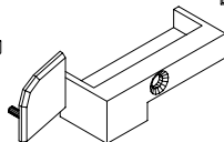
EŞİK ÜST PR. UÇ KAPAMA PARÇASI E399.211
