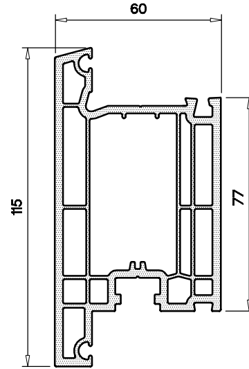
DIŞA AÇILAN KAPI-115/4 PROFİLİ 1161.596
