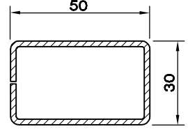
KUTU PR. ( 50 X 30 X 2.0 ) 5399.222
