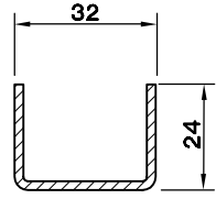
U DESTEK SACI ( 32 X 24 X 2.0 ) 5161.912
