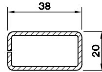
KUTU PR. ( 20 X 38 X 2.0 ) 5399.212
