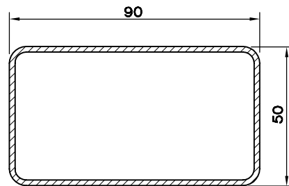
KUTU PR. ( 50 X 90 X 2.0 ) 5399.232
