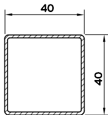
KUTU PR. ( 40 X 40 X 1.5 ) 5399.411
