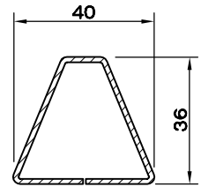
135° KÖŞE DÖNÜŞ DESTEK SACI ( 1.5 ) 5399.421
