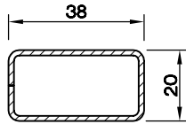
KUTU PR. ( 20 X 38 X 1.5 ) 5399.211
