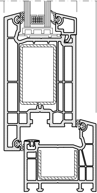
KESİT
