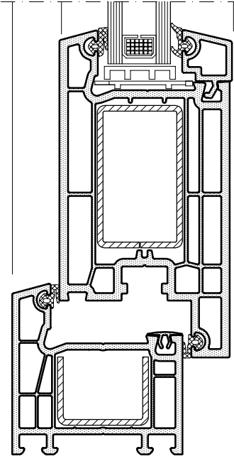
KESİT
