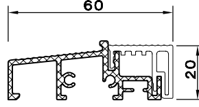
AL. EŞİK PR. 6399.103
