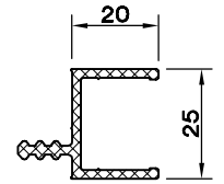
AL. PARAPET ADAPTÖR PR. 6599.201
