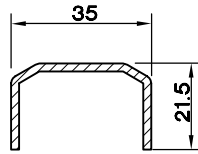
KANAT -50/3 DESTEK SAÇI (2.0) 5160.252
