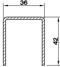
U DESTEK SAÇI 36 X 42 (2.0) 5175.922
