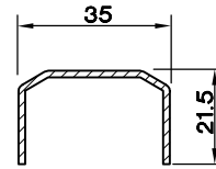
KANAT -50/3 DESTEK SAÇI (1.5) 5160.251
