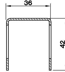
U DELİKLİ DESTEK SAÇI 36 X 42 (1.5) 5261.911
