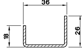
U DESTEK SAÇI 36 X 18 X 26 (2.0) 5175.912
