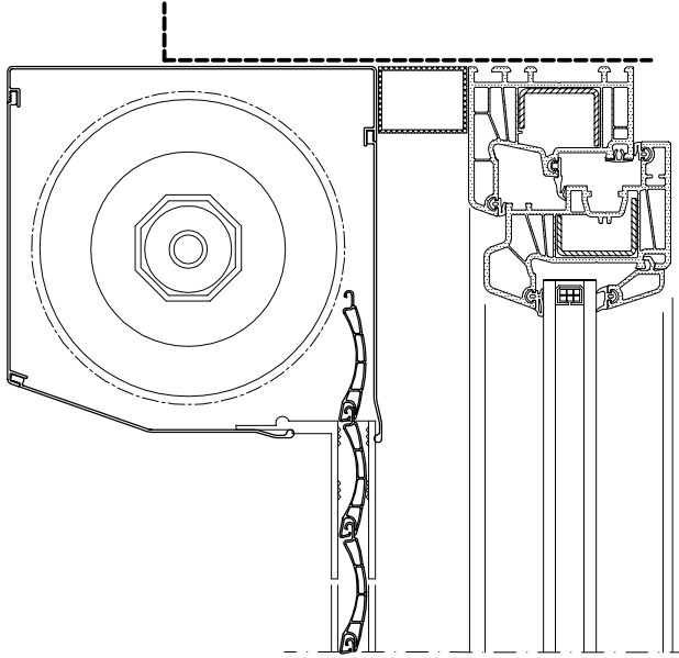
DOĐRAMAYA MONTAJLI
