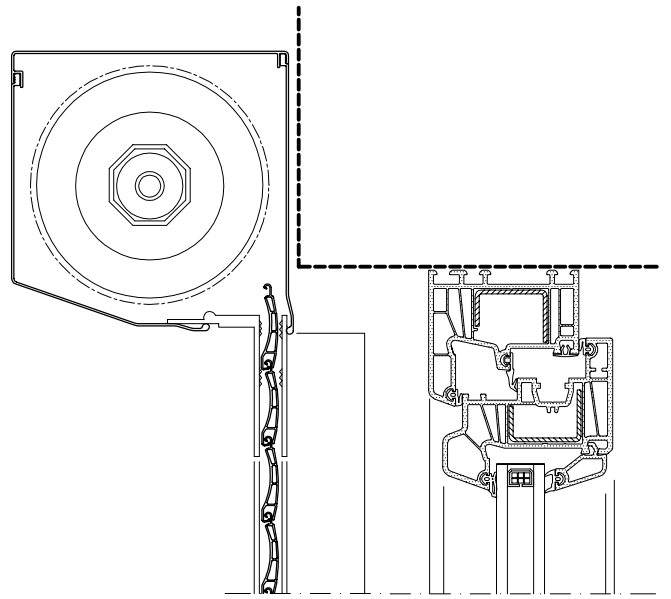
DUVARA MONTAJLI
