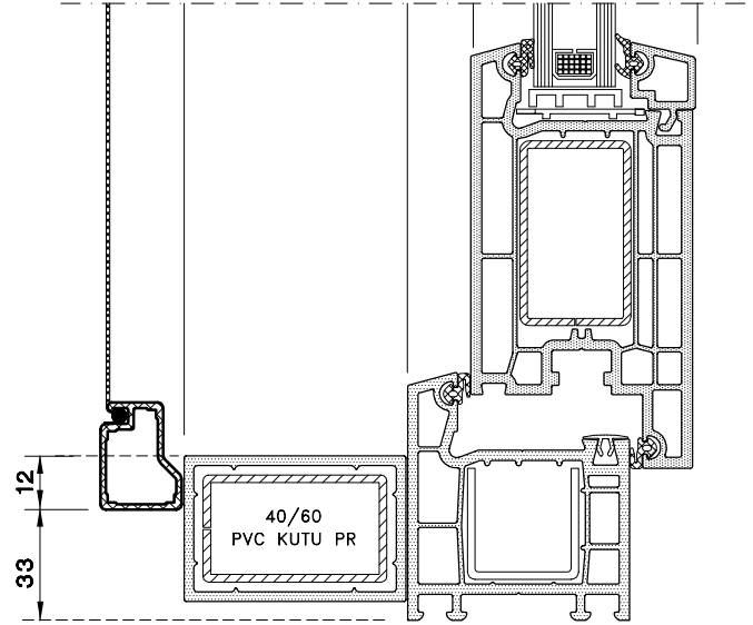
KESİT
