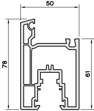
GENİŞ KANAT - 50 PROFİLİ 11S1.250
