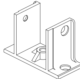
ORTAKAYIT BAĞLAMA PARÇASI 51S7.511
