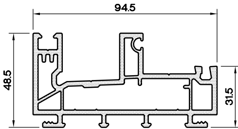
SABİT BÖLMELİ KASA - 95 PROFİLİ 11S2.195
