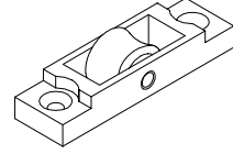
DAR KANAT TEKERLEĞİ H1S2.111
