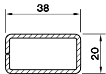
KUTU PR. ( 20 X 38 X 2.0 ) 5399.212
