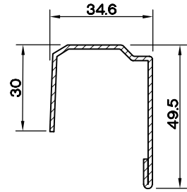
GENİŞ KANAT -50 DESTEK SACI (1.5) 51S7.211
