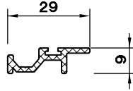
AL. ARA SIZDIRMAZLIK PR. 6399.407
