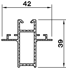
AL. SÜRME KİLİTLEME PR. 6399.405
