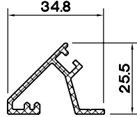
AL. KÖŞE DÖNÜŞ PR. 6399.409
