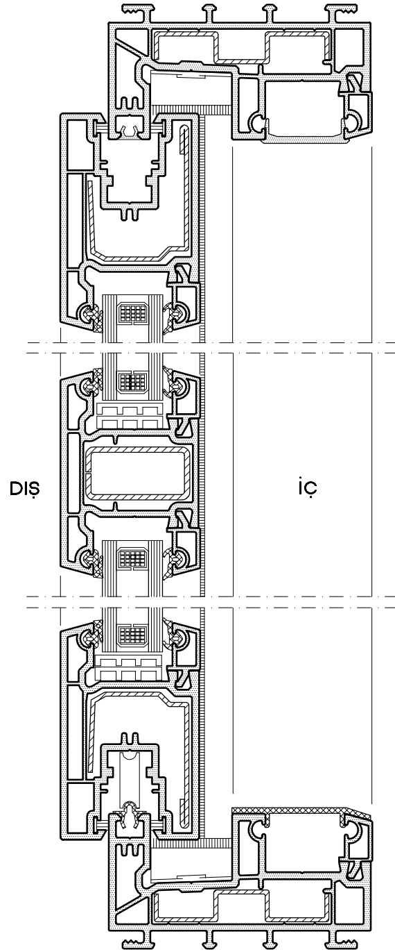
KESİT
